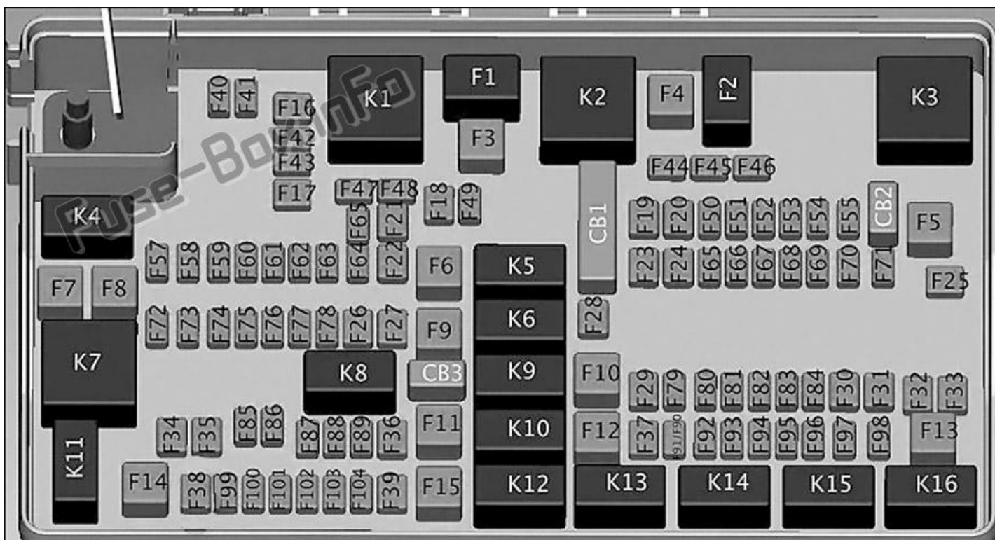
Zuordnung der Sicherungen (2014)
